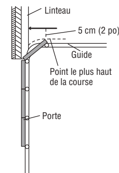
Porte articulée avec guide courbé
